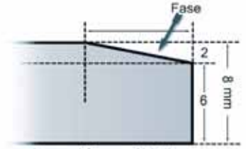
Fasenskizze: gilt für alle Modelle
